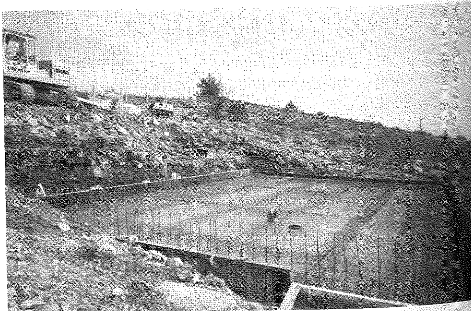
Le chantier du nouveau réservoir
